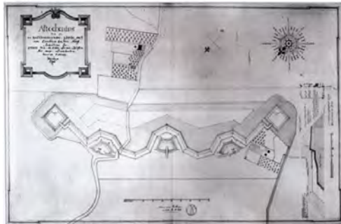
Een 'Afteekening van de gebastioneerde linie ... in plaats van de Oude Linie Buijten Het dorp Linschoten. Voor de Vesting Woerden. 1796'. (MvC)
